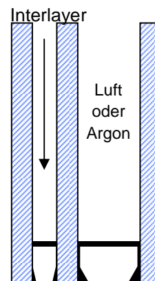
Iso-Aufbau für die Außenanwendung
